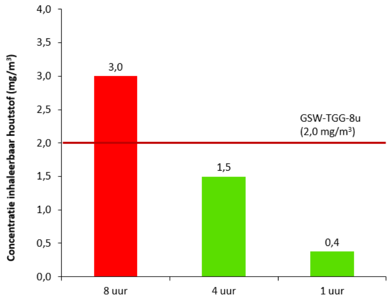
Figuur 2 . Toetsing blootstelling inhaleerbaar houtstof aan grenswaarde
