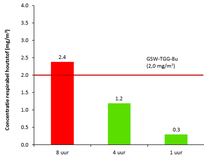
Figuur 1. Toetsing blootstelling inhaleerbaar houtstof aan grenswaarde
