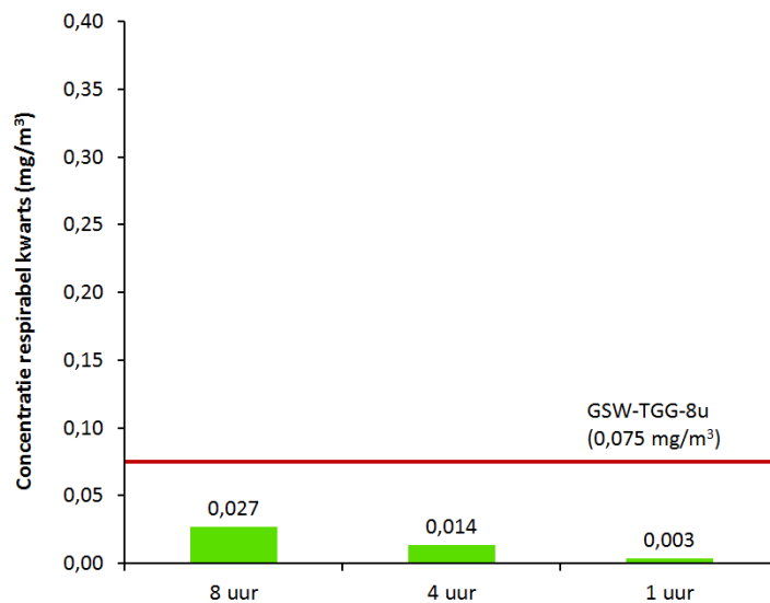
Figuur 1 . Toetsing blootstelling respirabel kwarts aan grenswaarde
