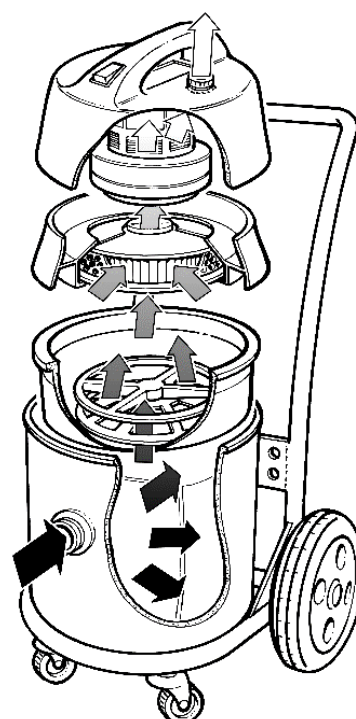
Figuur 2. Schematische weergave stofzuiger (HSE, 2017)
